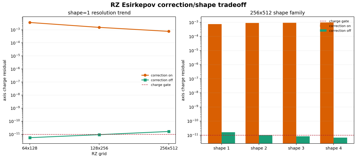
图 5-3: RZ Esirkepov axis-correction/shape tradeoff。左侧是 \text{shape}=1 的三档分辨率趋势, 右侧是 256x512 下 \text{shape}=1/2/3/4 的 correction-on/off 对照; 红色虚线是 1e-11 charge gate。所有 field gate 均通过, 但 correction-on 的 axis residual 仍约为 0(1e-3) , correction-off 的 charge 结果随 shape 变化, 不能据此修改全局默认值或宣称正式收敛阶。
