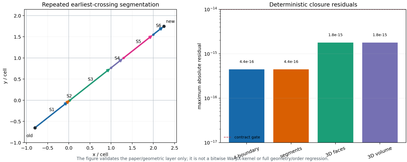
图 5-1: Villasenor 公式合同的两层证据。左侧把一条跨越多个 cell 的轨迹按 earliest crossing 切成局部 segment; 右侧汇总总边界、segment、3D face 和 3D volume closure 的最大残差。该图只展示论文/几何层闭合, 不把它升级为 WarpX kernel 等价或全 geometry/order 回归。
