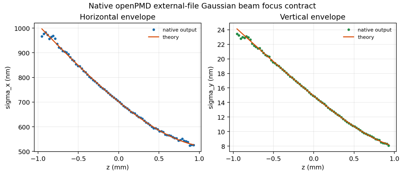
图 8-10 由 scripts/plot_gaussian_beam_focus_contract.py 从对应的 Gaussian beam 输出重新生成。
