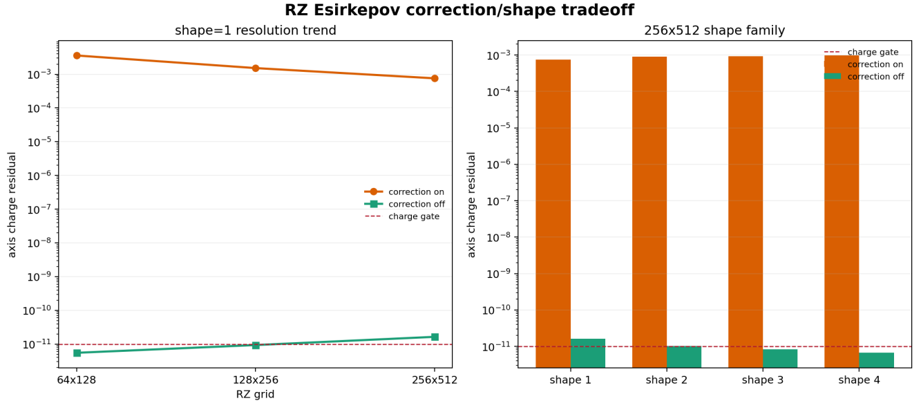
图 5-3: RZ Esirkepov axis-correction/shape tradeoff。左侧是 shape=1 的三档分辨率趋势，右侧是 256x512 下 shape=1/2/3/4 的 correction-on/off 对照；红色虚线是 1e-11 charge gate。所有 field gate 均通过，但 correction-on 的 axis residual 仍约为 0(1e-3) ，correction-off 的 charge 结果随 shape 变化，不能据此修改全局默认值或宣称正式收敛阶。
