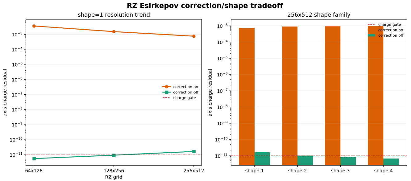
图 5-3: RZ Esirkepov axis-correction/shape tradeoff。左侧是 shape=1 的三档分辨率趋势, 右侧是 256x512 下 shape=1/2/3/4 的 correction-on/off 对照; 红色虚线是 1\text{e-}11 charge gate。所有 field gate 均通过, 但 correction-on 的 axis residual 仍约为 0(1\text{e-}3) , correction-off 的 charge 结果随 shape 变化, 不能据此修改全局默认值或宣称正式收敛阶。
