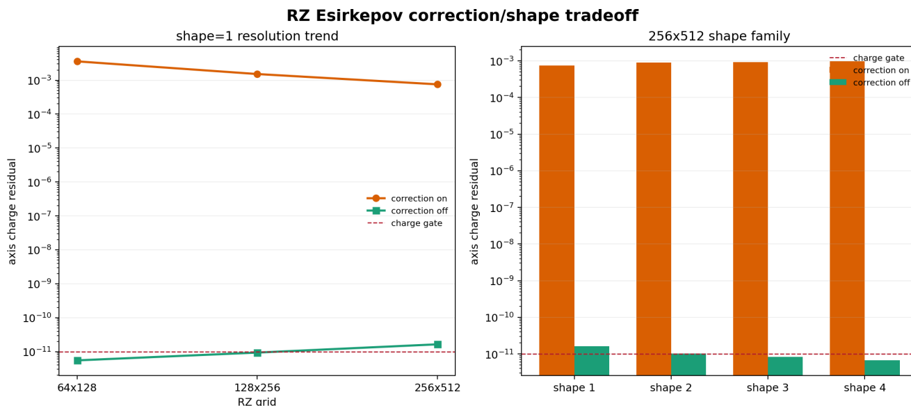
图 5-3: RZ Esirkepov axis-correction/shape tradeoff。左侧是 \text{shape}=1 的三档分辨率趋势, 右侧是 256x512 下 \text{shape}=1/2/3/4 的 correction-on/off 对照; 红色虚线是 1\text{e-}11 charge gate。所有 field gate 均通过, 但 correction-on 的 axis residual 仍约为 0(1\text{e-}3) , correction-off 的 charge 结果随 shape 变化, 不能据此修改全局默认值或宣称正式收敛阶。
