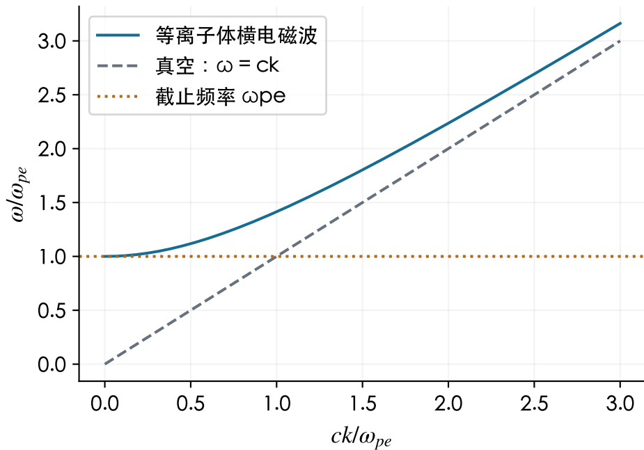
(a) 传播波有最低频率
