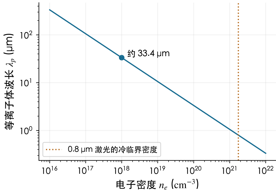
(a) 密度越高，电子响应尺度越短
