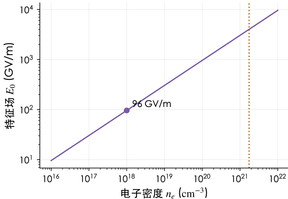
(b) 场更强不等于终能量更高
