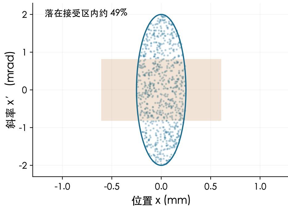
(b) 较小束斑、较大发散
