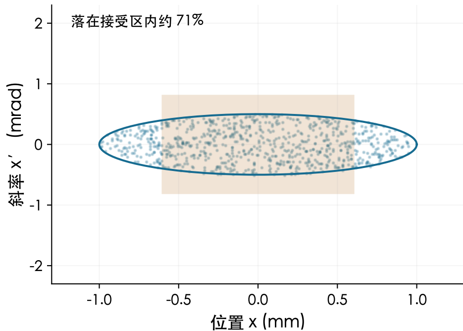
(a) 较大束斑、较小发散
