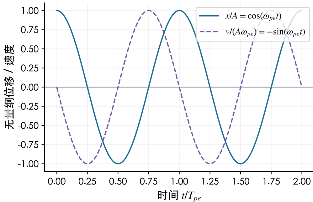
(b) 位移与速度相差四分之一周期
