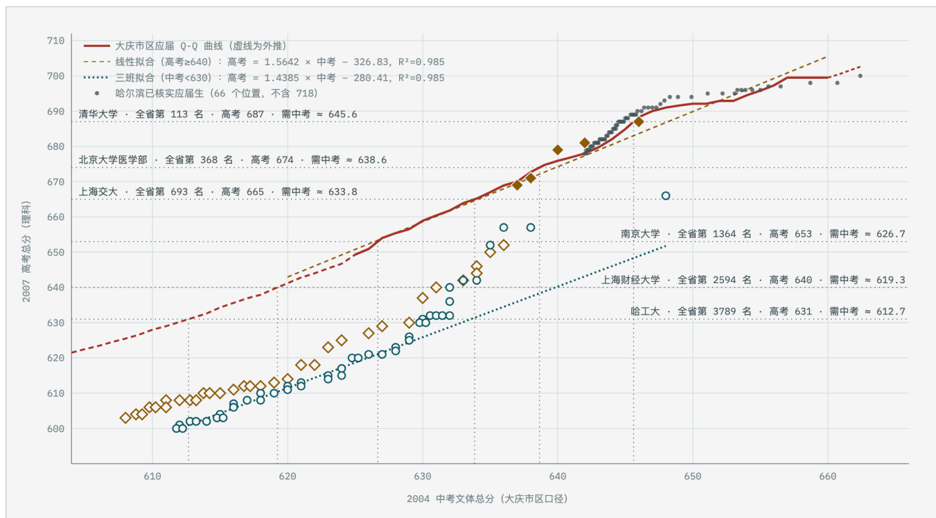
绥化一中高三三班 (蓝圈)、高三一班 (棕菱) 和哈尔滨市应届 (蓝色实点) 2004 年中考和 2007 年高考分位数-分位数图, 红线为大庆市区应届的对应曲线 (虚线为外推)
