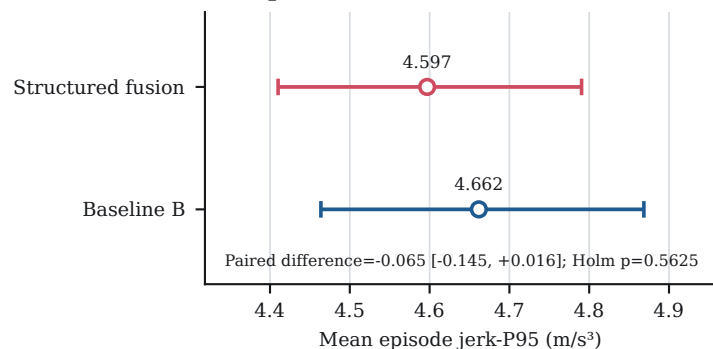
(d) Episode kinematic smoothness
