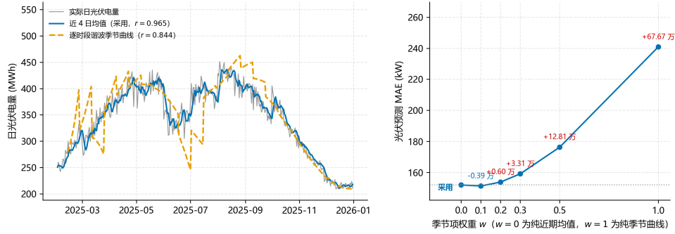
图 7 (a) 日光伏发电量与季节曲线对比；(b) 光伏 MAE 随季节曲线权重 w 的变化
