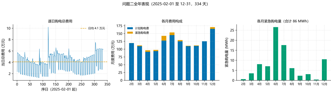
图 9 问题二全年表现：逐日购电总费用（左，虚线为日均值）、各月费用构成（中）、各月紧急购电量（右）
