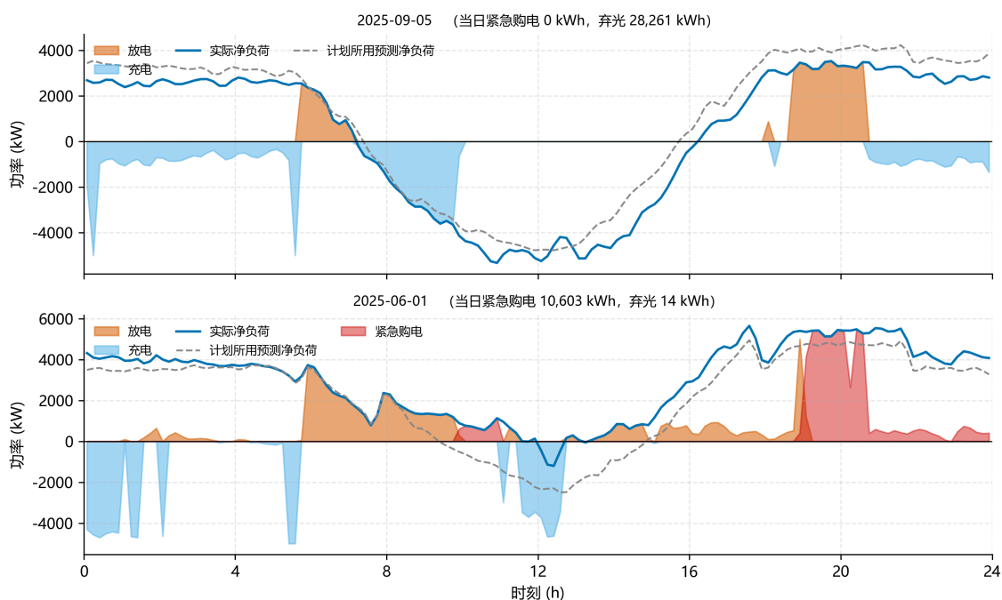
图 11 因果实时平衡控制过程：上行（2025-09-05）实际低于计划、储能吸收富余并出现弃光；下行（2025-06-01）实际高于计划、储能兜底后仍出现紧急购电
