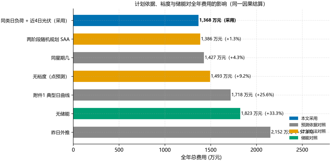
图 10 计划依据、安全裕度与储能对全年费用的影响（同一因果结算；蓝为采用方案）
