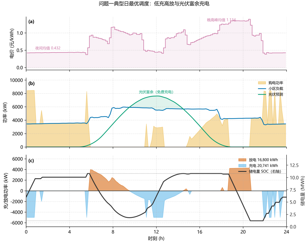
图 6 问题一典型日最优调度：电价、功率平衡、储能充放电与储电量
