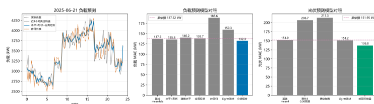
图 9 预测模型对照：分类组合负荷模型与岭回归堆叠光伏模型的精度优势
