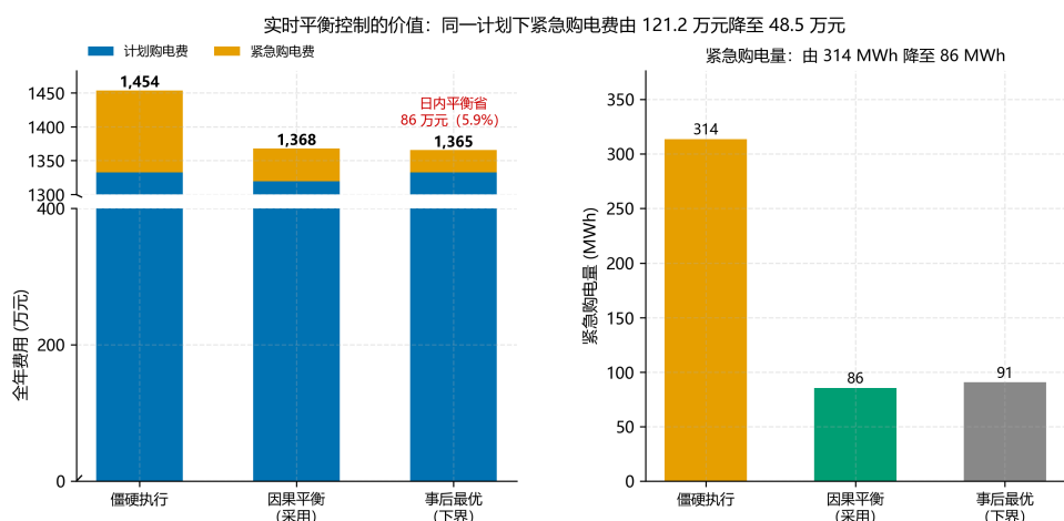
图 8 同一 0:00 计划下三种结算方式的费用分解（左，因计划购电费几乎相同而采用纵轴断轴）与紧急购电量（右，单位 MWh）：实时平衡控制把紧急购电费由 121.2 万元压到 48.5 万元
