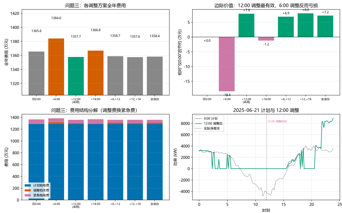
图 12 问题三：各调整方案全年费用（左上）、调整的边际价值（右上）、费用结构分解（左下）、2025-06-21 计划与逐段调整（右下）
