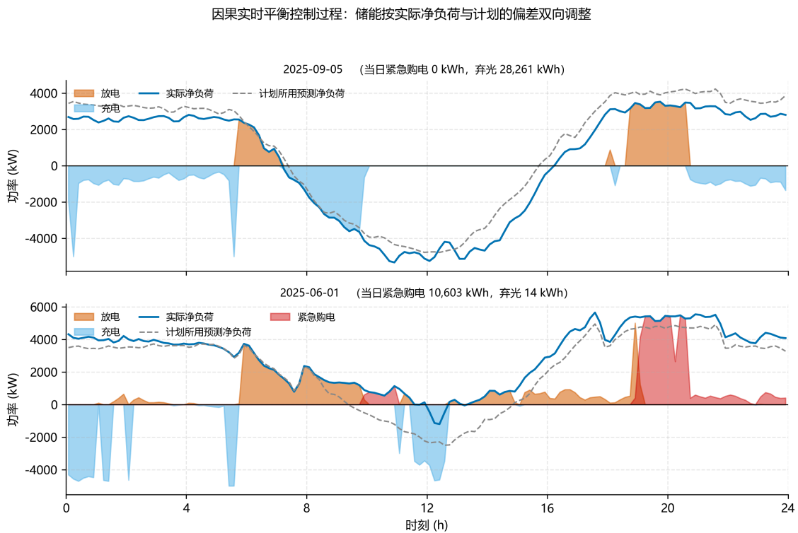
图 11 因果实时平衡控制过程：上行（2025-09-05）实际低于计划、储能吸收富余并出现弃光；下行（2025-06-01）实际高于计划、储能兜底后仍出现紧急购电
