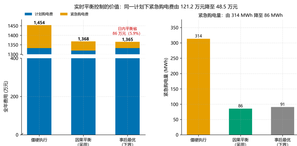
图 7 同一 0:00 计划下三种结算方式的费用分解（左，因计划购电费几乎相同而采用纵轴断轴）与紧急购电量（右，单位 MWh）：实时平衡控制把紧急购电费由 121.2 万元压到 48.5 万元
