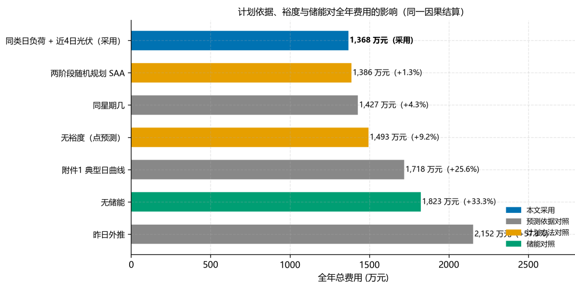
图 9 计划依据、安全裕度与储能对全年费用的影响 (同一因果结算；蓝为采用方案)
