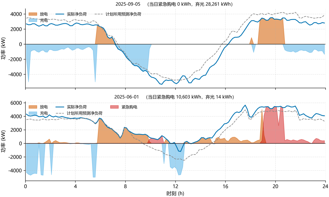
图 10 因果实时平衡控制过程：上行（2025-09-05）实际低于计划、储能吸收富余并出现弃光；下行（2025-06-01）实际高于计划、储能兜底后仍出现紧急购电
