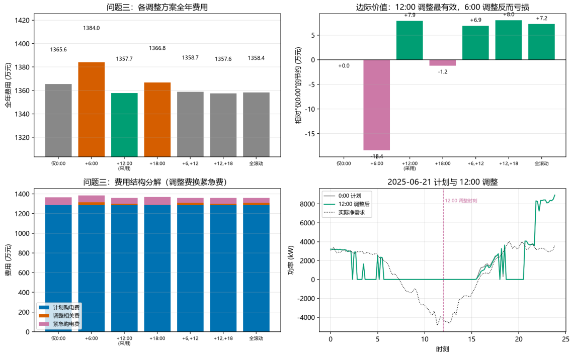
图 11 问题三：各调整方案全年费用（左上）、调整的边际价值（右上）、费用结构分解（左下）、2025-06-21 计划与逐段调整（右下）
