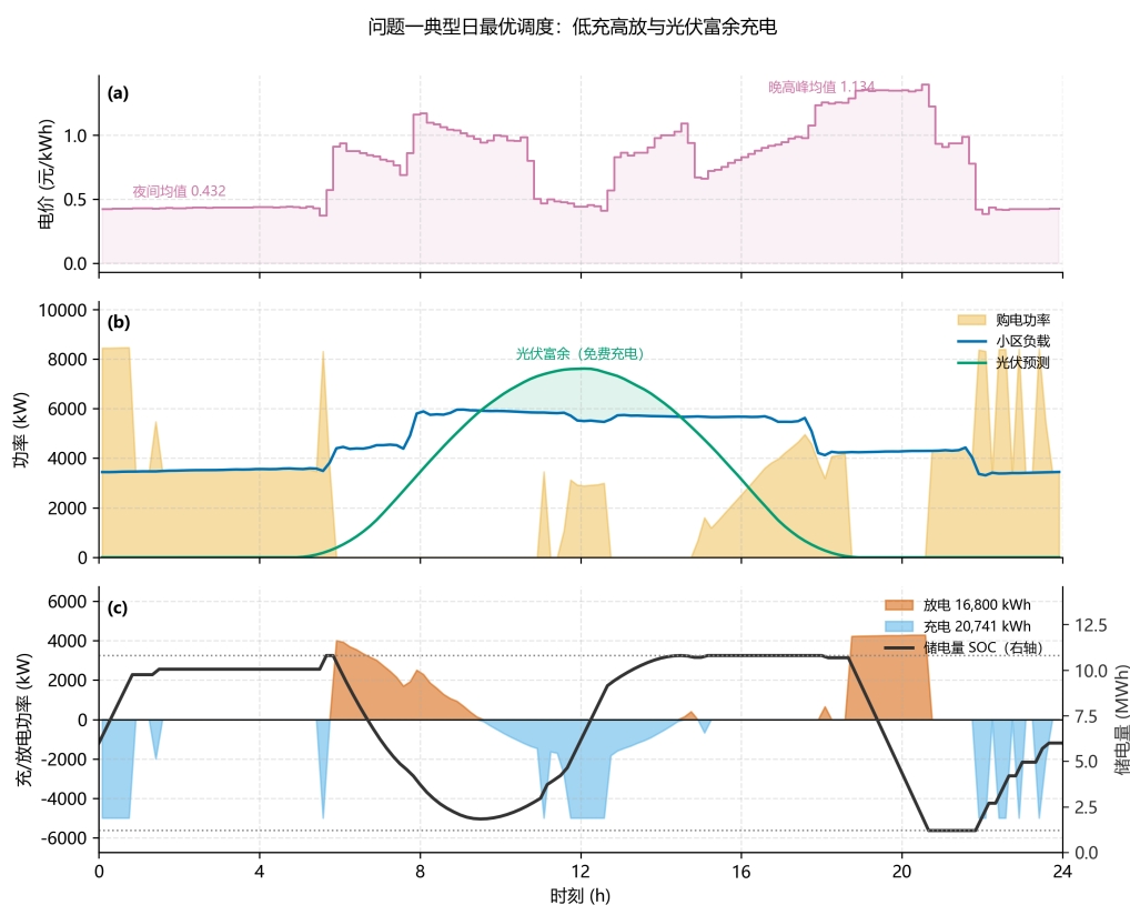
图 6 问题一典型日最优调度：电价、功率平衡、储能充放电与储电量
