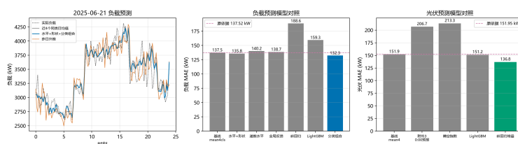
图 9 预测模型对照：分类组合负荷模型与岭回归堆叠光伏模型的精度优势
