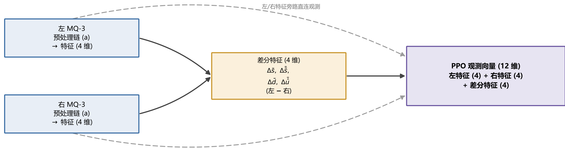
(b) 左右双传感器融合与 PPO 观测构造
