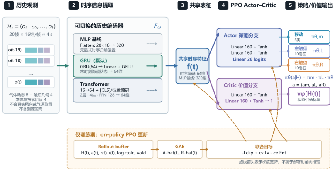
图 3-1 双触须主动嗅觉 PPO 的时序 Actor-Critic 网络架构。长度为 H = 20 的观测历史由每帧 16 维硬件可重建特征组成，不包含真实风向、气源位置或到源距离。历史编码器可在扁平 MLP、GRU 和 Transformer 之间切换，当前默认 GRU 将序列压缩为 64 维共享特征 f_t ；Actor 与 Critic 随后分别经过两层 160 单元全连接网络。Actor 的 26 个 logits 被拆分为移动 6 类、左触须 10 类和右触须 10 类三个分类分布，Critic 输出状态价值 v_\phi(\mathcal{H}_t) 。琥珀色虚线路径表示 rollout、GAE 与 PPO 联合目标对共享编码器及两条分支的训练期梯度更新，不属于部署时的前向推理路径。
