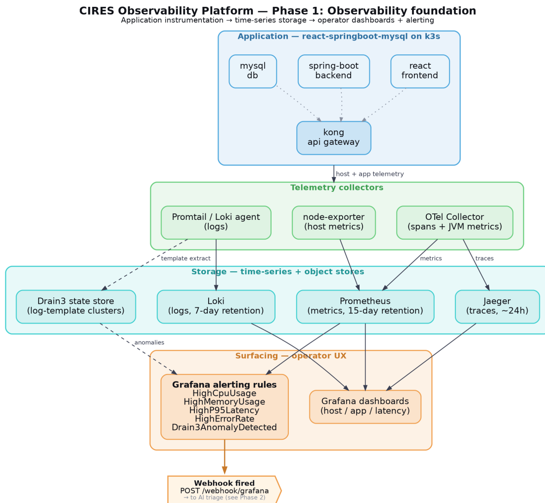
Figure 4.2. Phase 1 — fondation d’observabilité. L’instrumentation applicative (Spring Boot, Kong, MySQL, k3s) alimente les collecteurs (scrape Prometheus, Promtail, OTEL Collector) et le stockage (Prometheus TSDB, Loki, Jaeger). Grafana expose les données et achemine les alertes via le point de contact webhook de l’alerting unifié.
