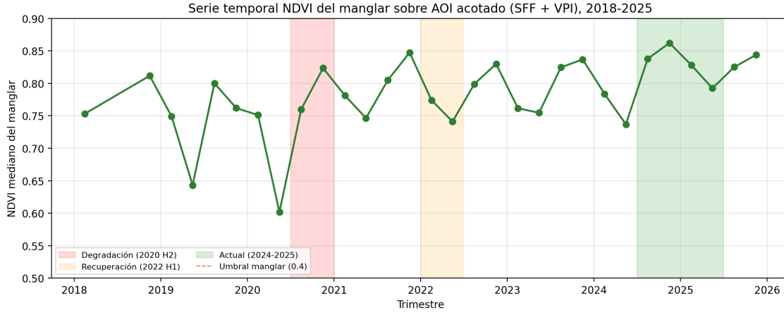
Figure 5: Serie temporal del NDVI mediaño del manglar sobre AOI acotado (SFF CGSM + VPI Salamanca, 835 km 2 ) entre 2018 y 2025, calculada a partir del datacube trimestral CF-1.8 restringida a píxeles con NDVI > 0,4 . Las franjas sombreadas marcan los tres periodos de referencia de la segmentación; la caída de 2019–2020 coincide con la sequía y el episodio La Niña que sostienen la narrativa del informe.
