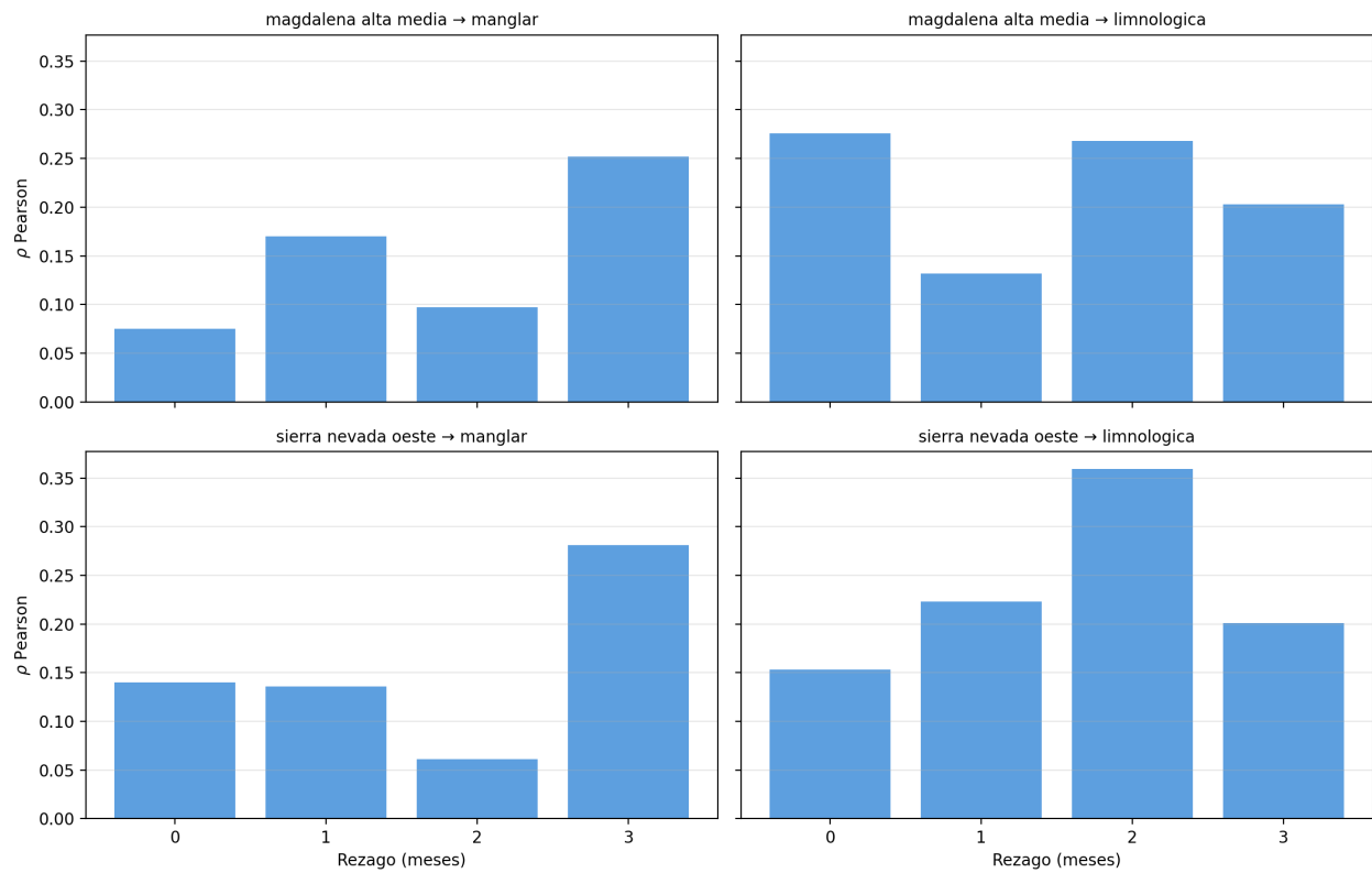
Figure 11: Correlación de Pearson entre anomalía mensual de precipitación CHIRPS y anomalía NDVI z-score de la CGSM, organizada por cuenca aportante (filas) y naturaleza espectral del sitio de monitoreo (columnas), con rezagos temporales de cero a tres meses. La convergencia con la figura equivalente del caudal IDEAM (figura Figure 9) ofrece doble validación de la dirección y magnitud del acoplamiento hidroclimático sobre el manglar.
