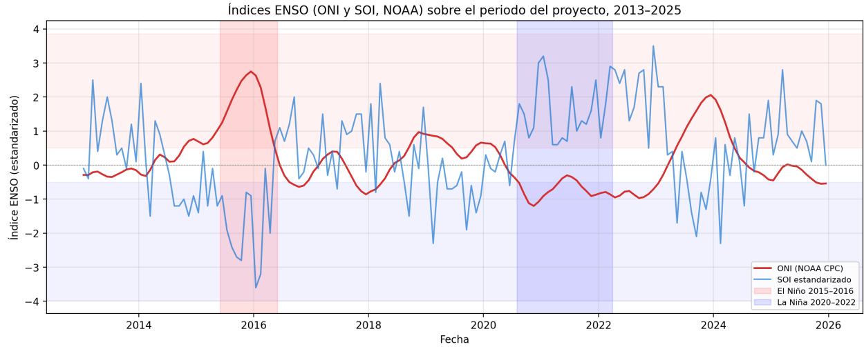
Figure 6: Índices ENSO mensuales (ONI y SOI, Climate Prediction Center de la NOAA) sobre el periodo del proyecto 2013–2025. Las franjas sombreadas marcan los dos eventos ENSO documentados: El Niño 2015–2016 que sostiene los quiebres bfast del periodo medio del análisis y La Niña 2020–2022 que sostiene la mortandad del manglar de septiembre 2020.
