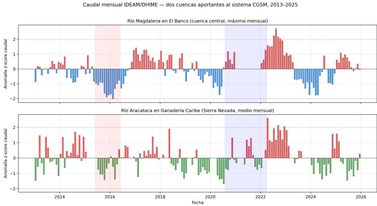
Figure 8: Series temporales de anomalía z-score del caudal mensual IDEAM para el río Magdalena en El Banco (panel superior, máximo mensual) y el río Aracataca en Ganadería Caribe (panel inferior, medio mensual), 2013–2025. Las franjas sombreadas marcan los dos eventos ENSO documentados; nótese que los picos de caudal extremo ( z > +2 ) ocurren en 2022, no en 2020.
