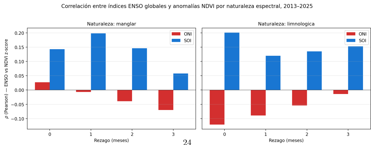
Figure 7: Correlación entre los índices ENSO globales (ONI en rojo, SOI en azul) y las anomalías NDVI z-score, desagregada por naturaleza espectral de las estaciones, para rezagos de cero a tres
