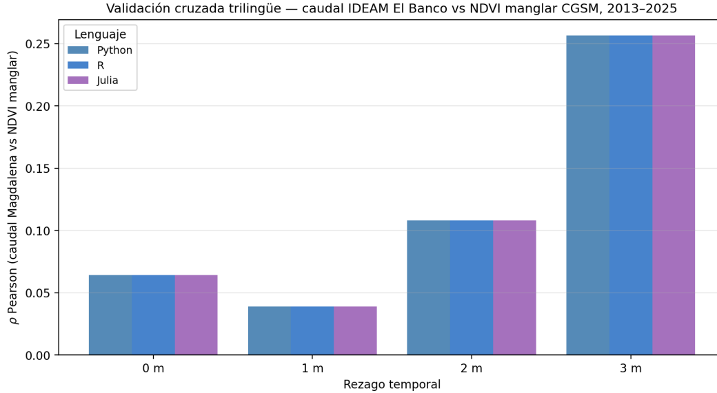
Figure 12: Validación cruzada trilingüe Python + R + Julia sobre la correlación de Pearson entre el caudal medio mensual del río Magdalena en El Banco y la anomalía NDVI z-score de las cuatro estaciones de manglar de la CGSM, con rezagos de cero a tres meses, 2013–2025. Las tres barras de cada rezago son visualmente idénticas, de esta manera la convergencia numérica entre los tres lenguajes hasta tres decimales valida la independencia del análisis respecto al entorno computacional.
