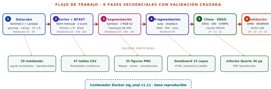
Figure 4: Flujo metodológico del proyecto: seis fases secuenciales con validación cruzada entre Python, R y Julia, todas ejecutadas dentro de un contenedor Docker que garantiza la reproducibilidad bit a bit de cada análisis.
