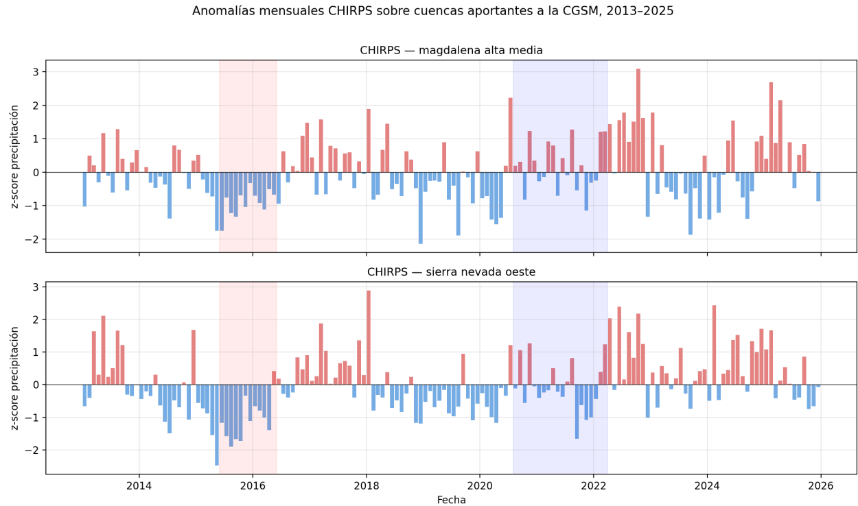
Figure 10: Anomalías mensuales de precipitación CHIRPS sobre las dos cuencas aportantes a la CGSM —cuenca alta-media del Magdalena (panel superior) y vertiente occidental de la Sierra Nevada (panel inferior)—, 2013–2025. Las franjas sombreadas marcan El Niño 2015–2016 (con anomalías negativas sostenidas que confirman la sequía documentada) y La Niña 2020–2022 (con dominancia de anomalías positivas que confirman el régimen húmedo). Los picos extremos z > +2 se concentran en 2022, en línea con la observación equivalente sobre los caudales IDEAM (figura Figure 8).
