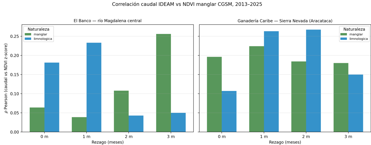
Figure 9: Correlación de Pearson entre anomalía de caudal IDEAM y anomalía NDVI z-score, desagregada por estación hidrológica (paneles), naturaleza espectral del sitio de monitoreo (barras verdes manglar, azules limnológicas) y rezago temporal de cero a tres meses. Las correlaciones positivas universales reflejan el efecto beneficioso del aporte fluvial sostenido sobre la productividad del manglar.
