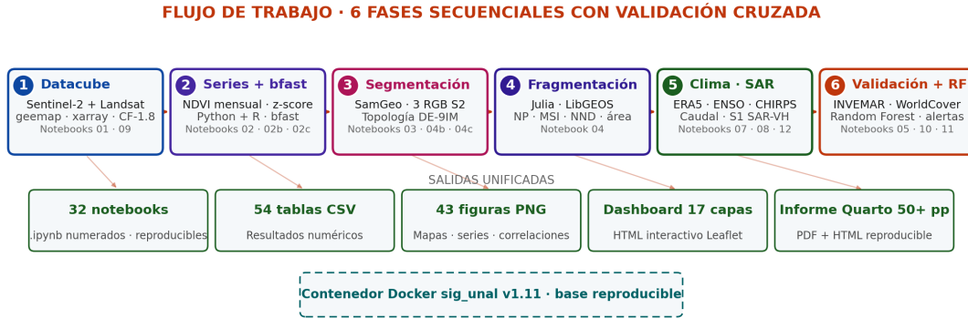
Figura 3: Flujo metodológico del proyecto: seis fases secuenciales con validación cruzada entre Python, R y Julia, todas ejecutadas dentro de un contenedor Docker que garantiza la reproducibilidad bit a bit de cada análisis.
