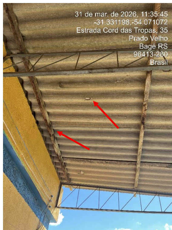
Figura 7: Telhas reparos e madeiramento com sinais de apodrecimento.
