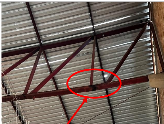
Fotos – Detalhes dados na tesoura metálica.
