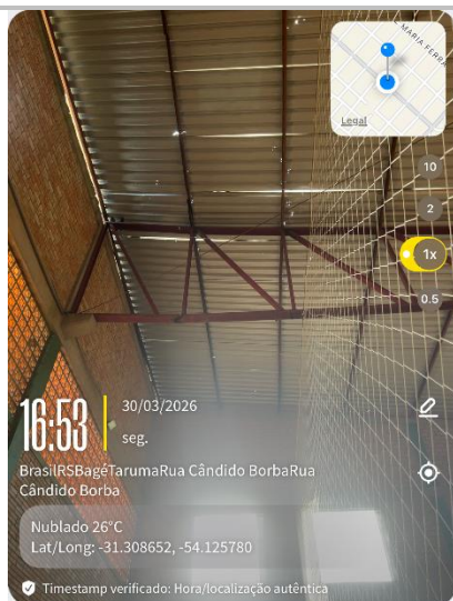
Fotos – Detalhes danos na cobertura – Tesoura e Telhas Metálicas
