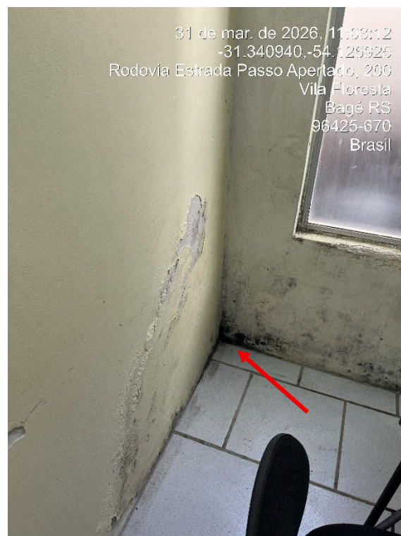
Figura 5: Infiltração no piso em decorrência do acúmulo de água.
