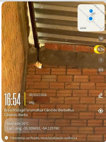
Fotos – Detalhes danos na cobertura – Tesoura e Terça.
