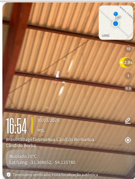
Fotos – Detalhes danos na cobertura - Telhas Metálicas
