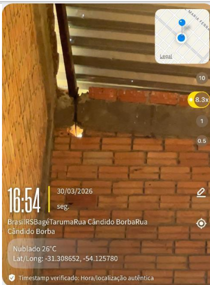
Fotos – Detalhes danos na cobertura – Tesoura (flambagem) e Terça.
