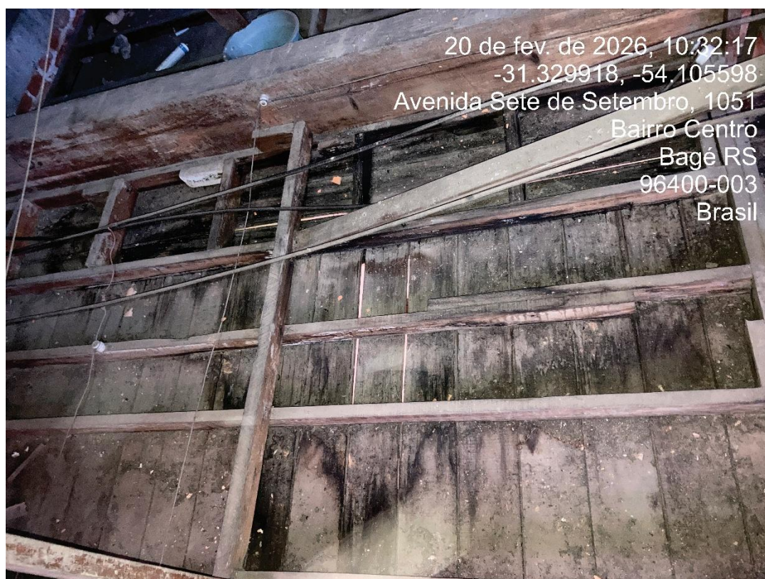
Figura 12: Forro danificado em decorrência de goteiras.
