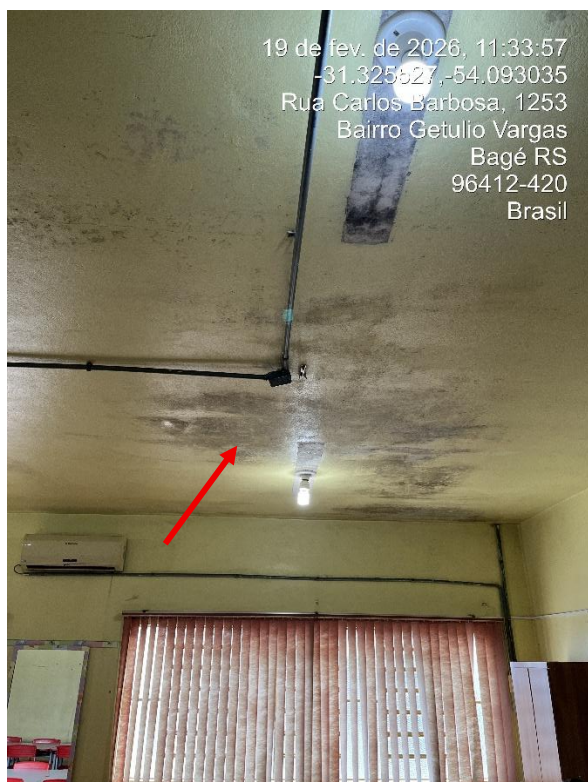
Figura 2: Presença de umidade na laje, próximo à rede elétrica.
