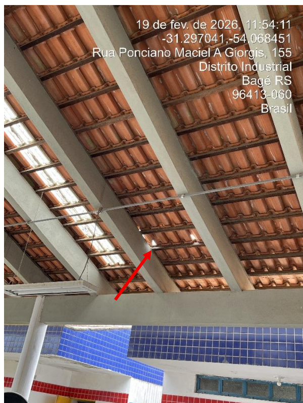
Figura 2: Telhas quebradas, evidenciando pontos de goteiras.
