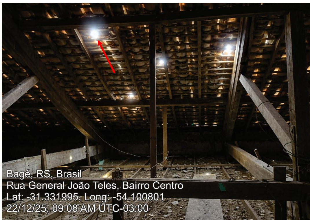
Figura 10: Estrutura de madeira que sustenta o telhado, evidenciando telhas quebradas.
