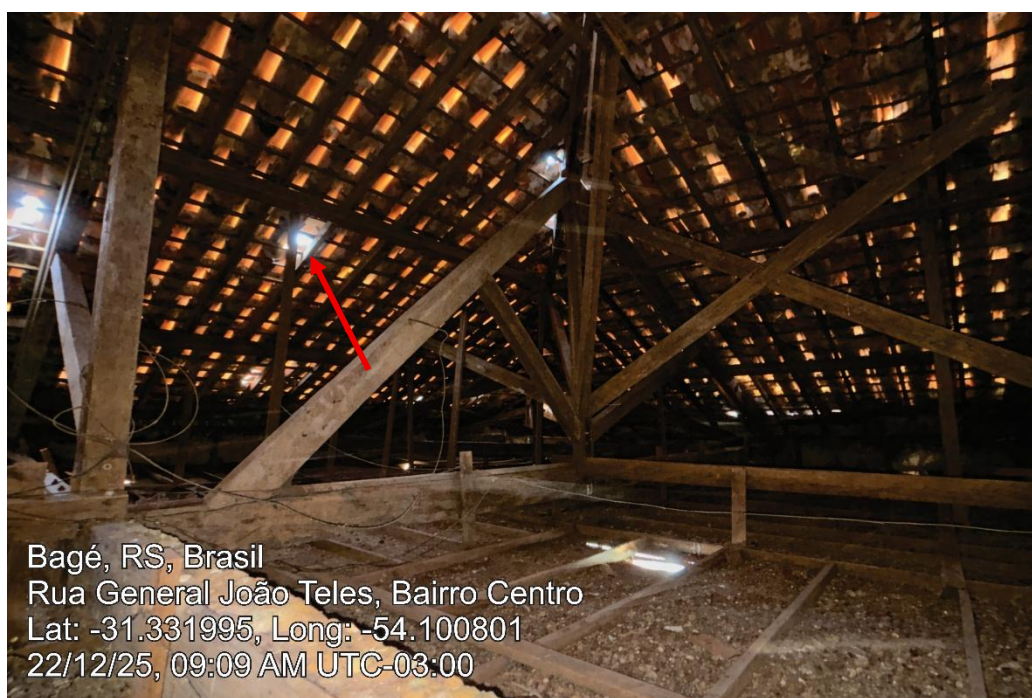
Figura 9: Estrutura de madeira que sustenta o telhado, evidenciando telhas quebradas.
