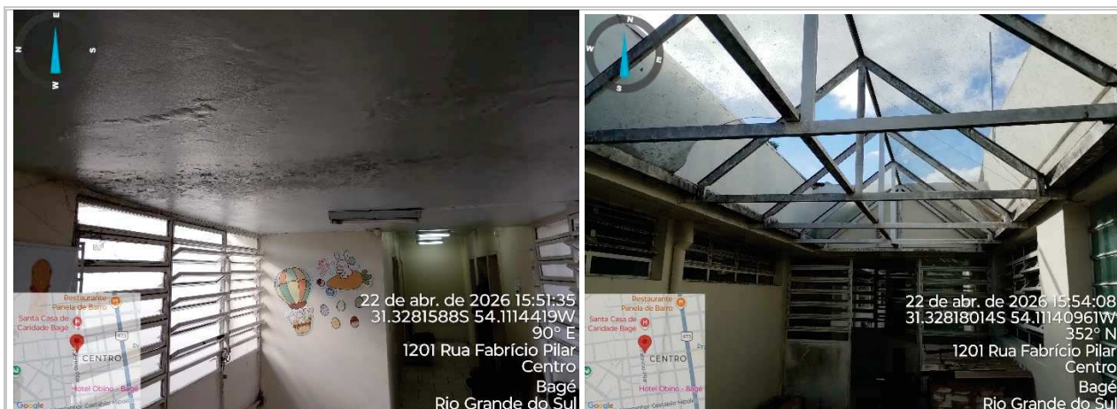
Fotos – Vista interna laje e estrutura de vidro.
