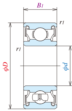
接触シール形 Contact sealed type DD
