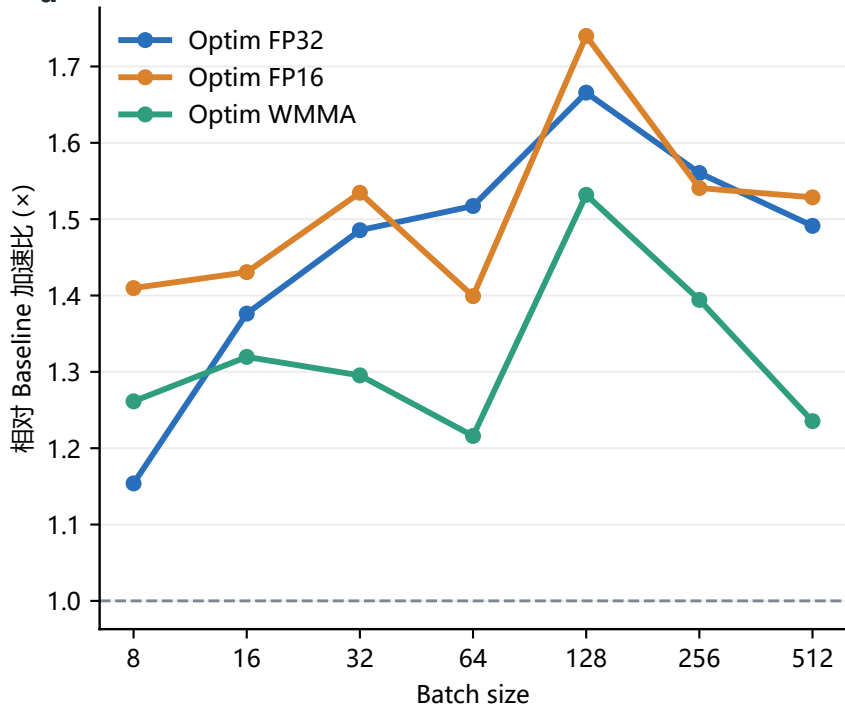
a 吞吐量加速比
