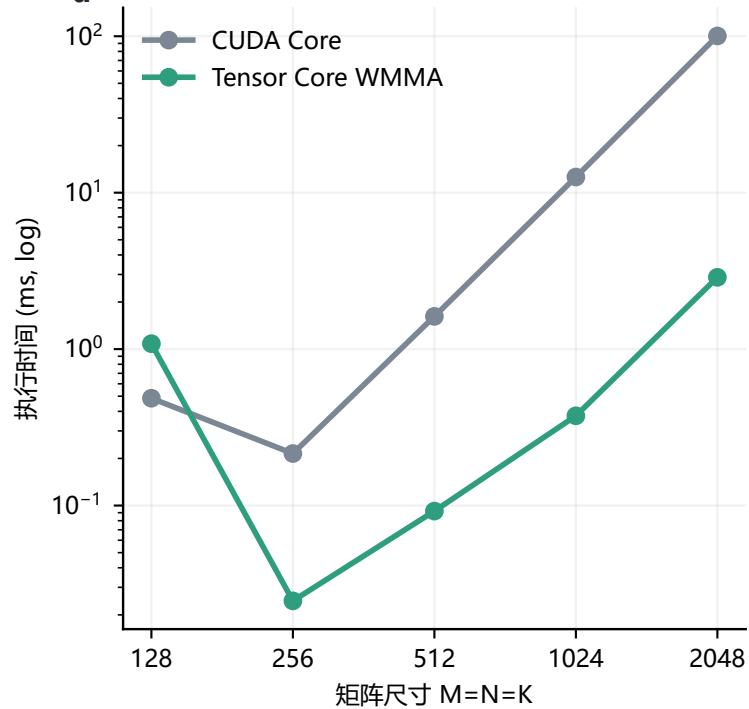
a FP16 GEMM 执行时间
