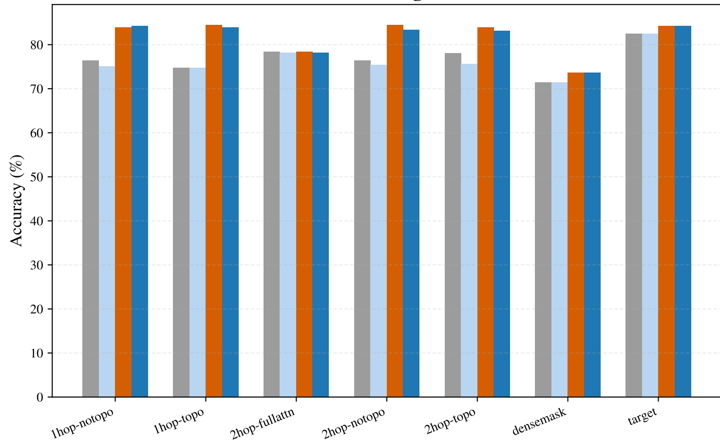
Cora Logit
