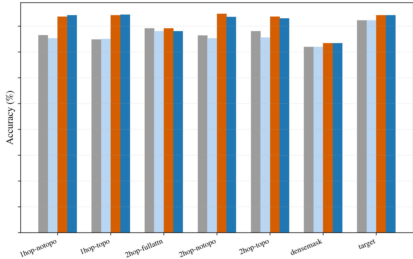
Cora Infill
