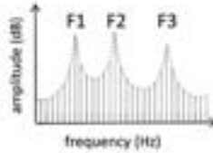
스펙트럼
