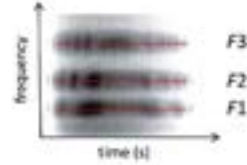
스펙트로그램
