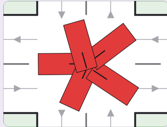
Collision: fan
