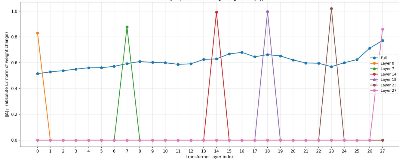
Per-layer parameter change magnitude ||\Delta||
