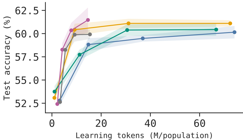
(b) GLM-5.3-Flash
