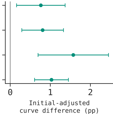
(b) GLM-5.3-Flash
