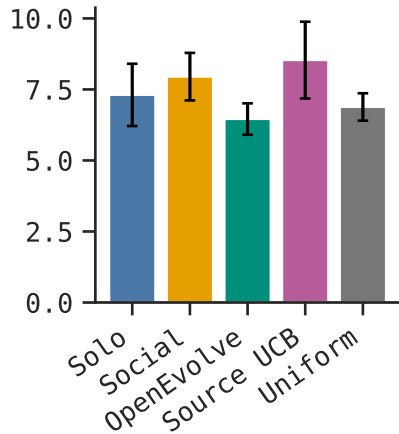
(d) GLM-5.3-Flash
