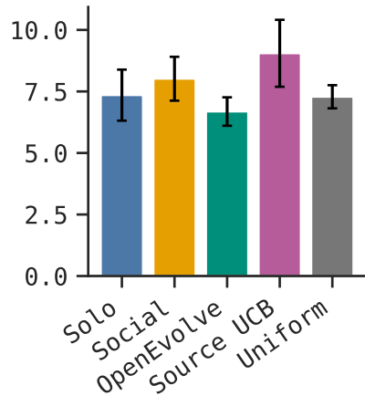
(b) GLM-5.3-Flash
