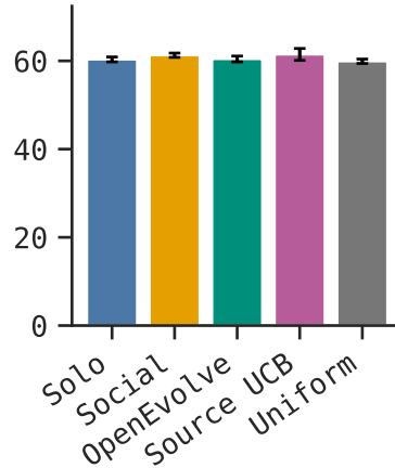
(d) GLM-5.3-Flash
