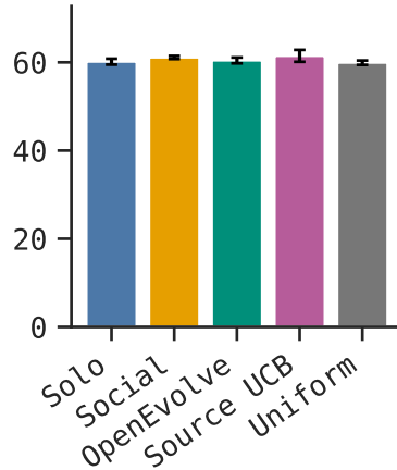
(b) GLM-5.3-Flash
