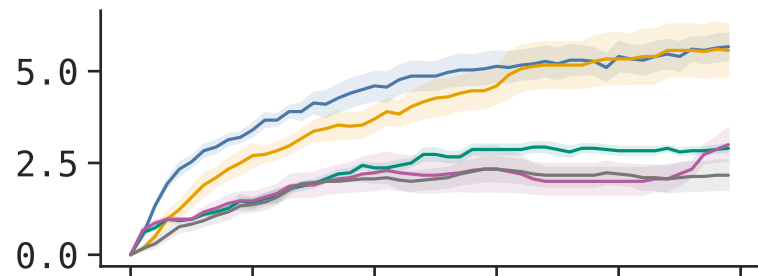
(b) GLM-5.3-Flash
