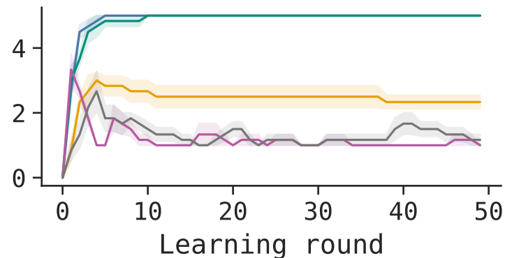
(f) GLM-5.3-Flash
