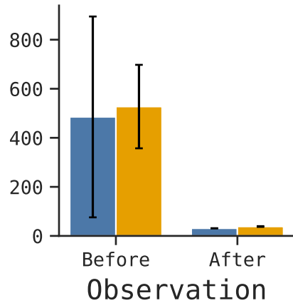
(d) GLM-5.3-Flash
