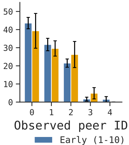
(b) GLM-5.3-Flash
