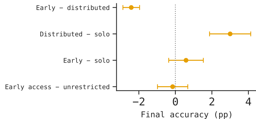
(b) GLM-5.3-Flash
