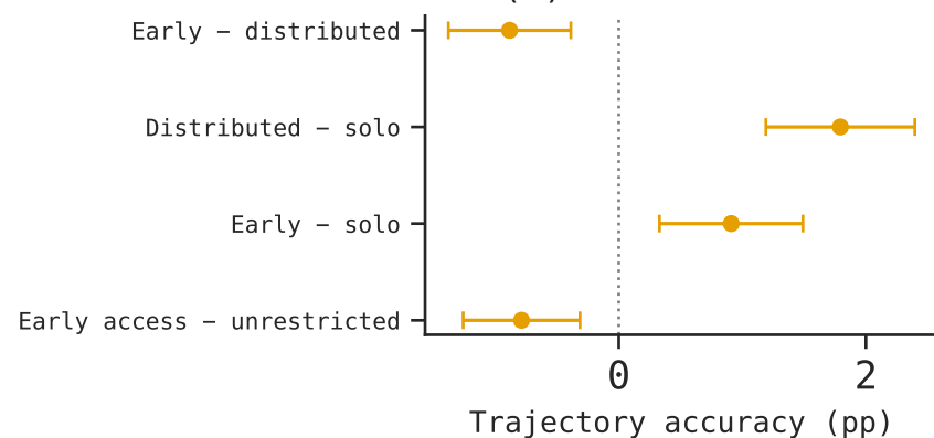
(d) GLM-5.3-Flash
