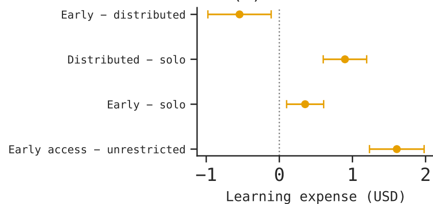
(f) GLM-5.3-Flash
