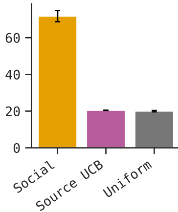
(d) GLM-5.3-Flash
