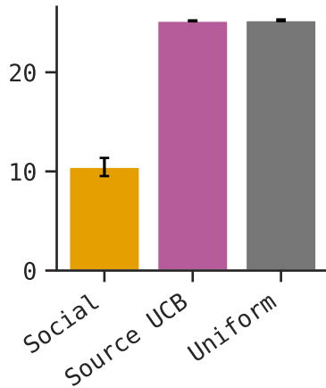
(b) GLM-5.3-Flash
