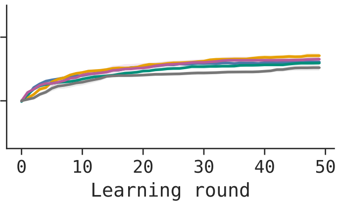
(b) GLM-5.3-Flash
