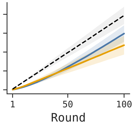
(b) GPT-OSS
