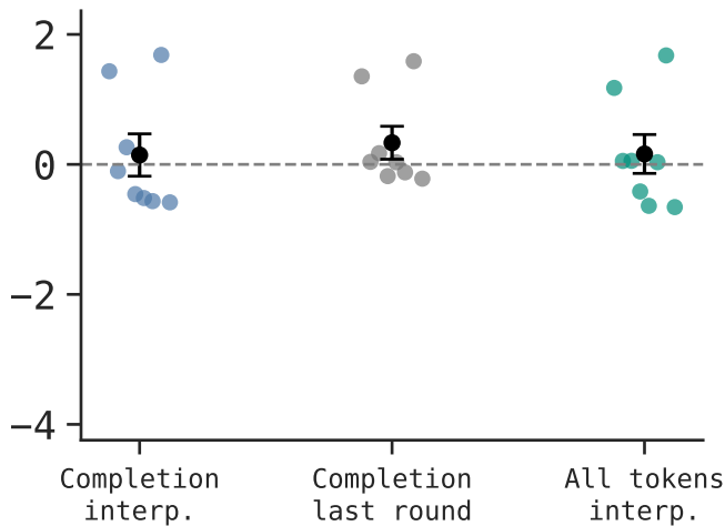
(a) Qwen3-14B
