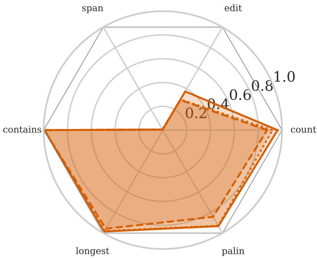
Gemma31 [NT]
