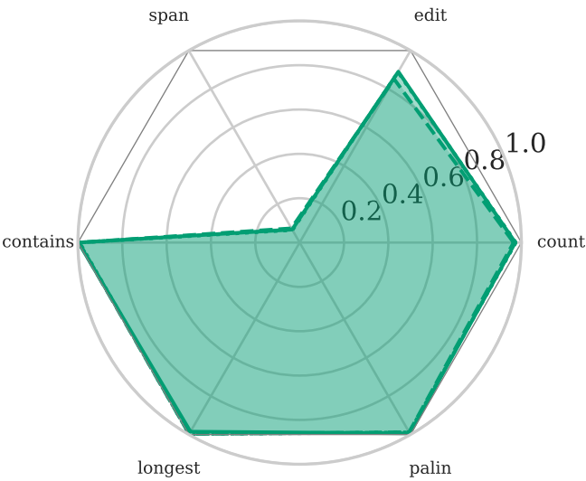
GPT-OSS20 [T]
