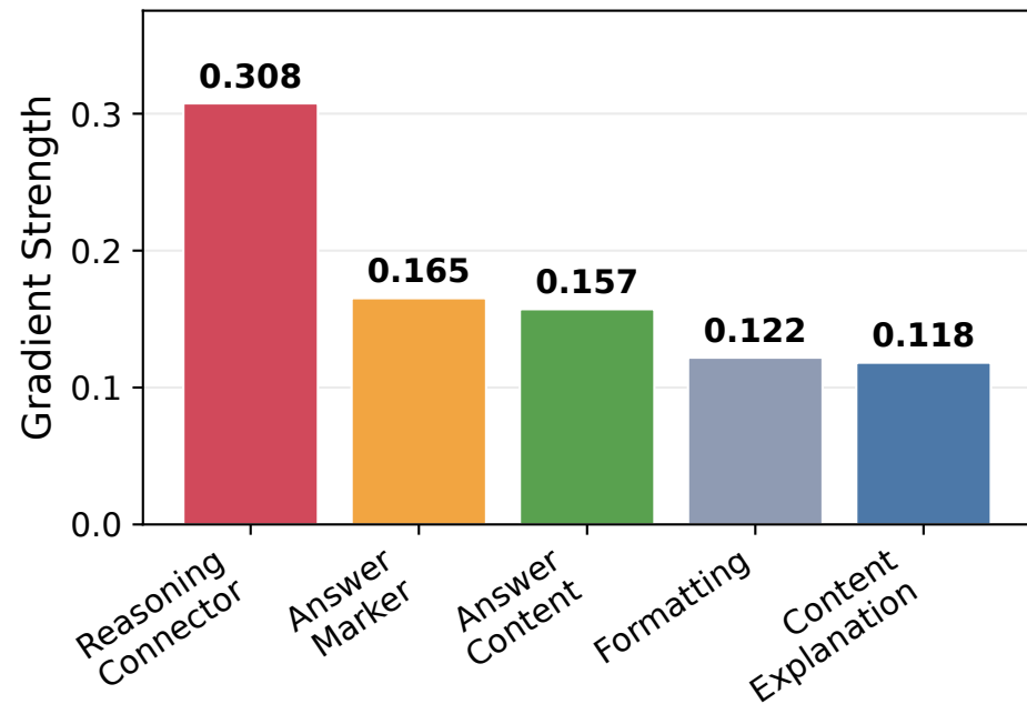
GPQA-Diamond
