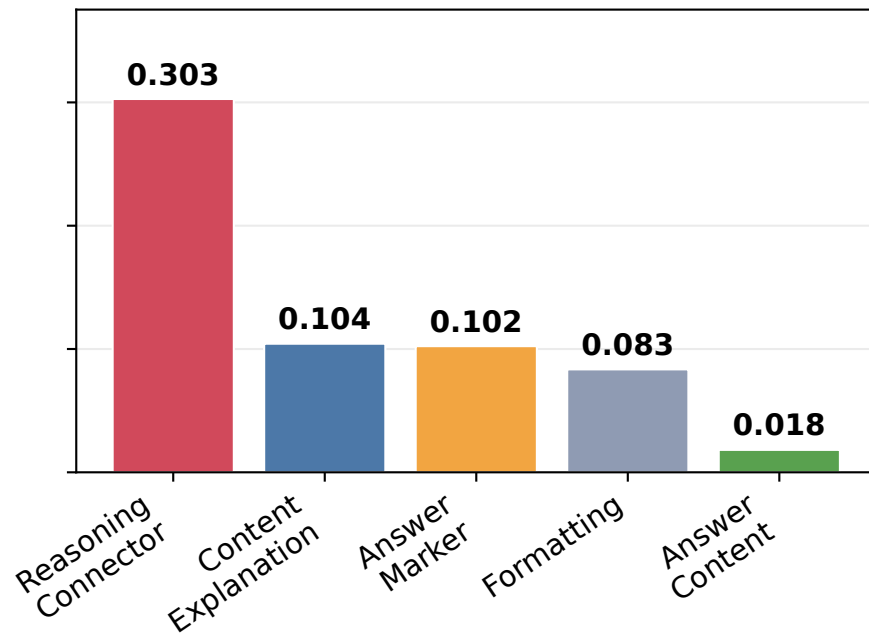
GSM8K
