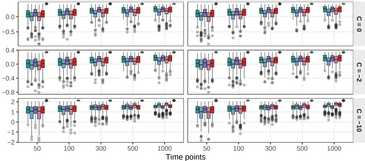
True PS
