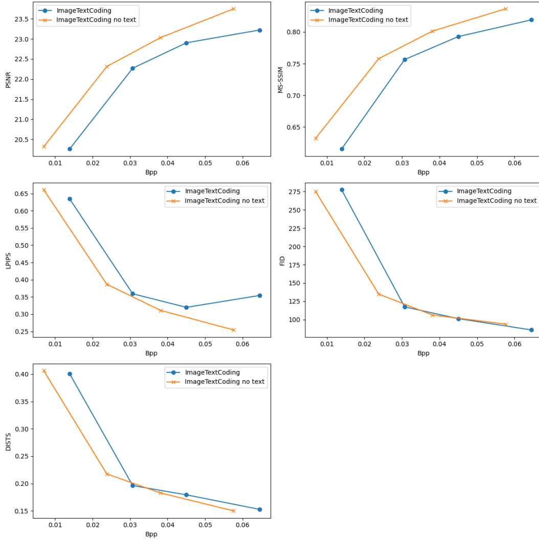
图 4 加和不加图像描述测试性能对比
