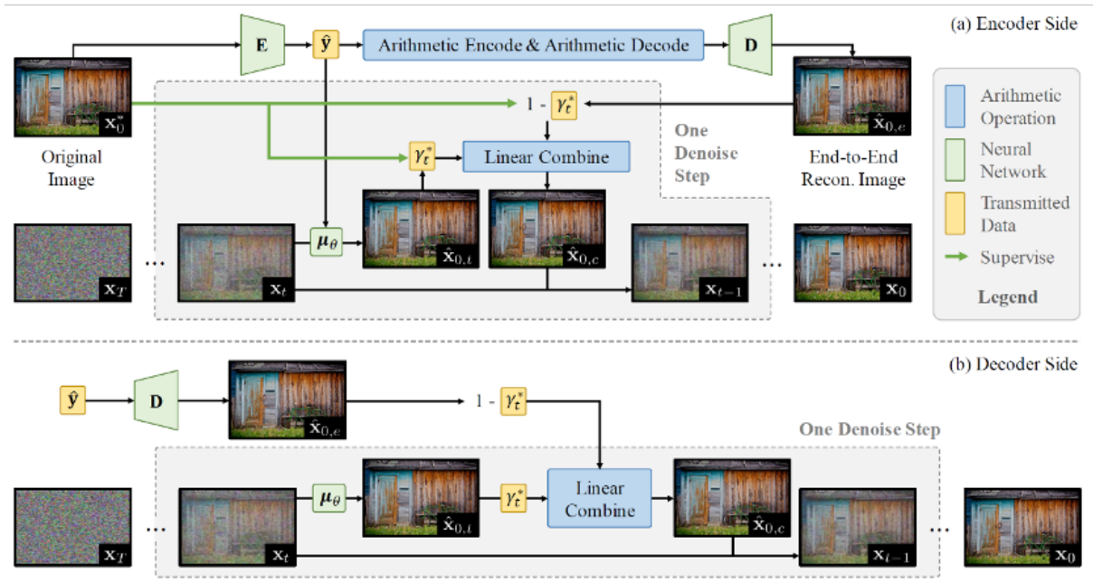
图 6 提案[VC-54-M466]模型结构示意图
