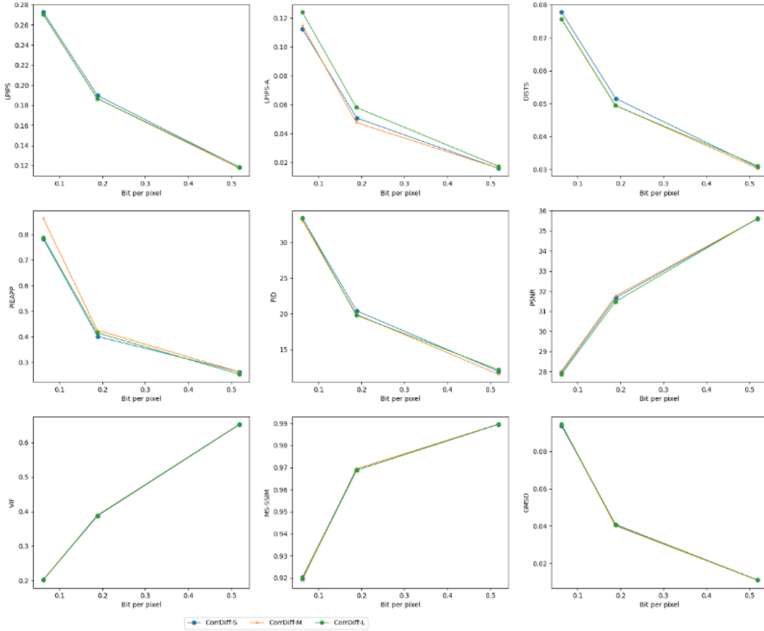
图 7 提案[VC-54-M466]模型在 CLIC 数据集上的评估结果
