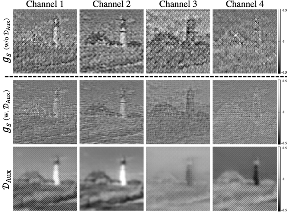
图 3 加和不加辅助解码器训练 StableCodec 在潜在空间上的对比示意图
