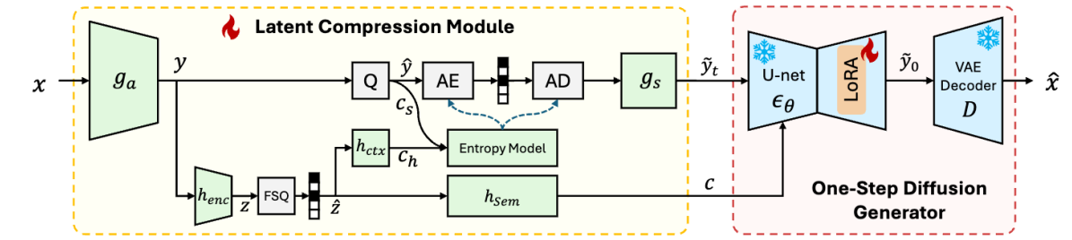
图 5 OneDC 模型结构示意图
