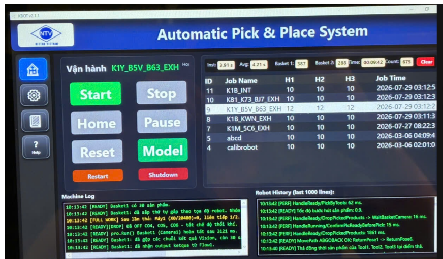
Hình 1. Nhóm nút vận hành chính trên màn hình Home
