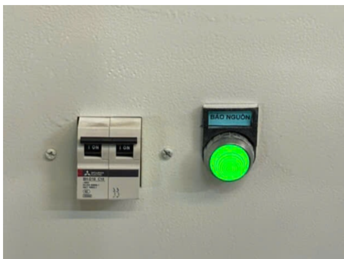
Hình 2. Aptomat nguồn và đèn BÁO NGUỒN trên tủ điều khiển
